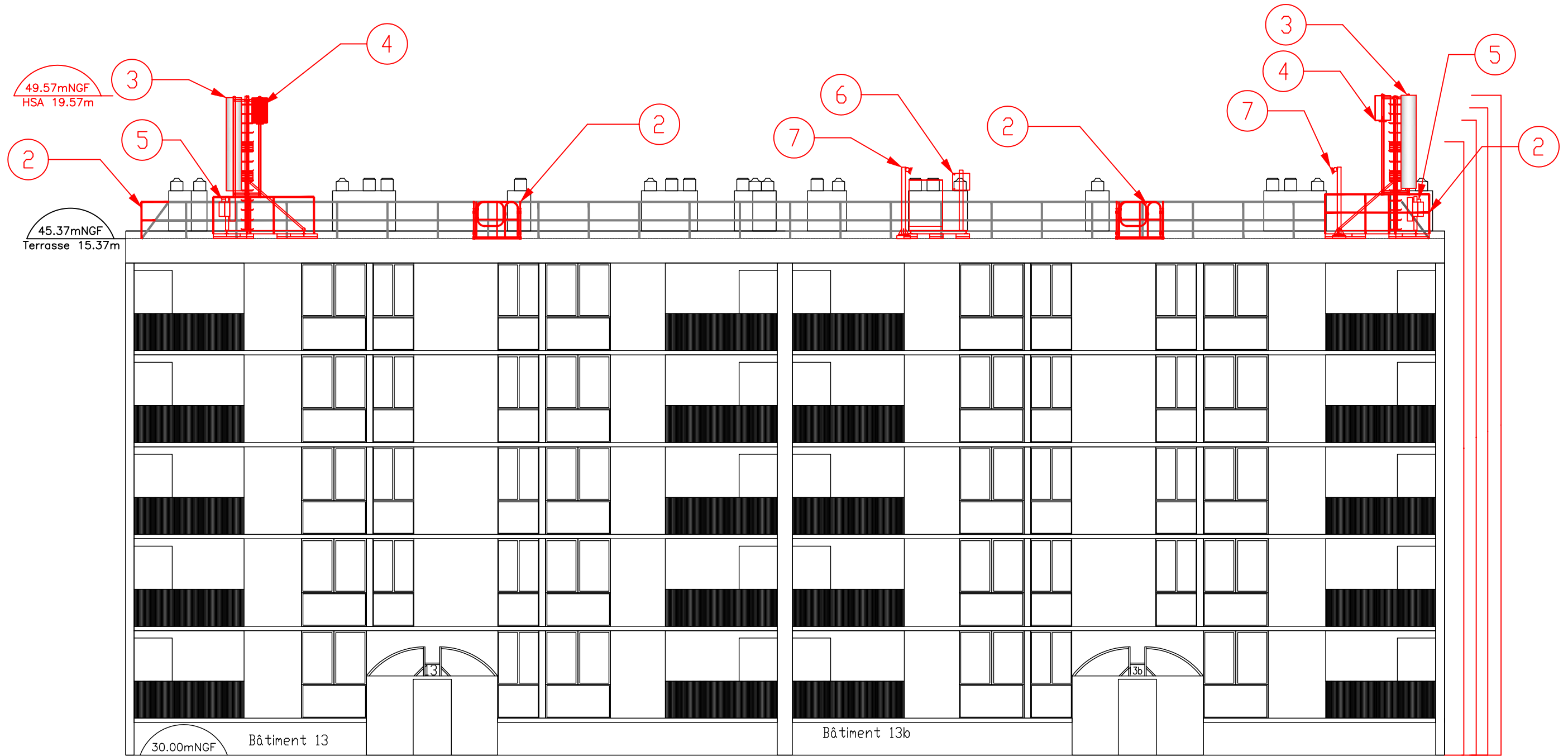
Elevation Nord-Ouest
